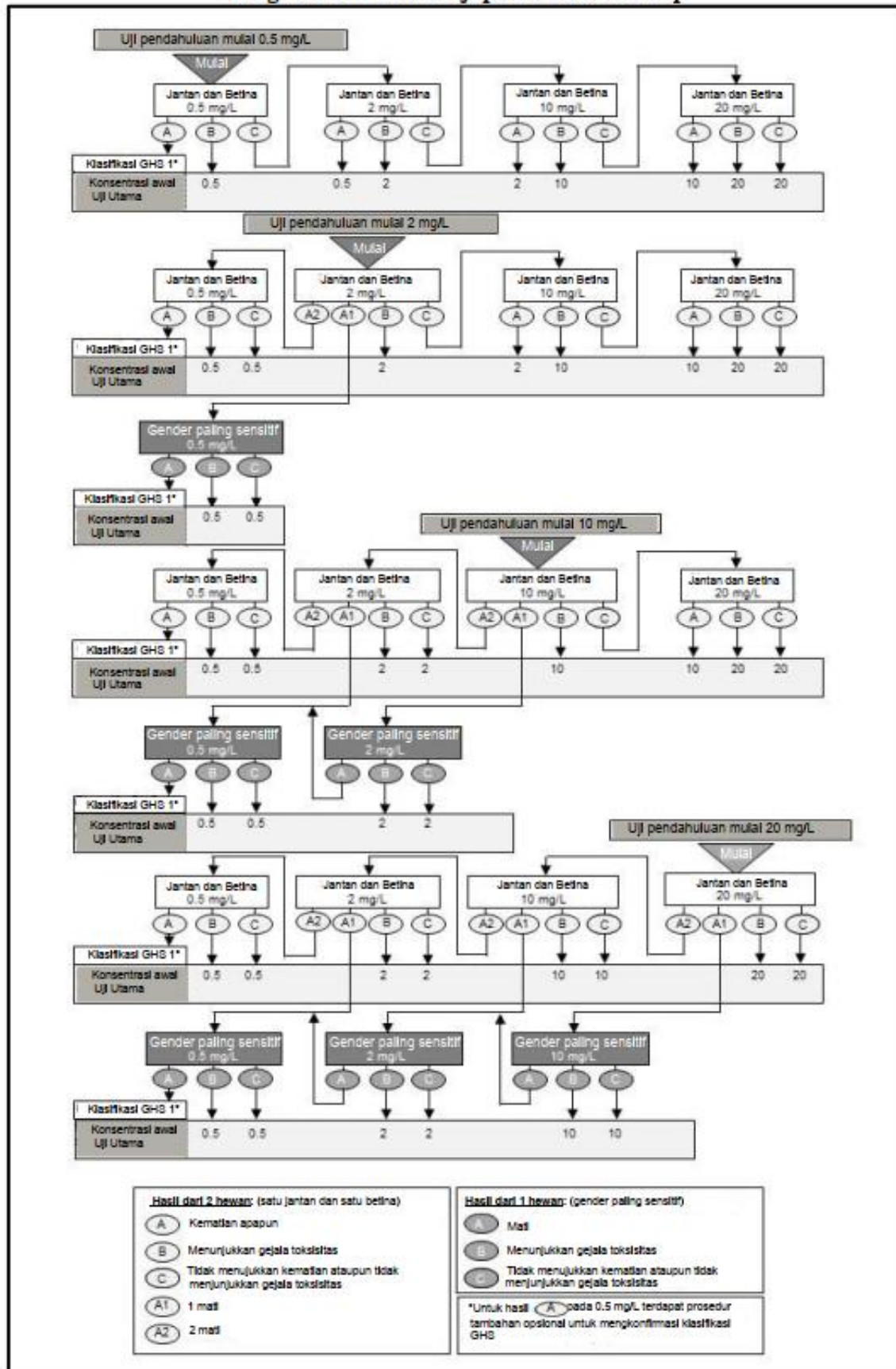
Diagram alir untuk uji pendahuluan - uap
